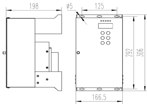
图 1-2 变频器外形及安装尺寸说明（单位 mm）
