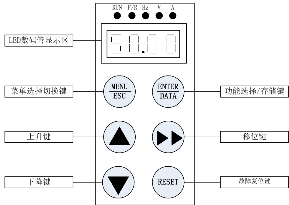
图3-1 操作面板（键盘）示意图
