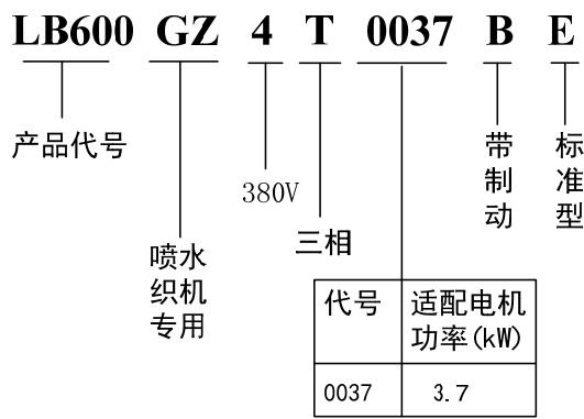
图1-1 变频器的型号
