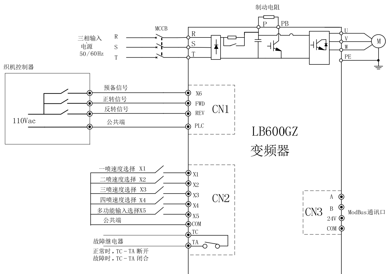
图 2-1 LB600GZ 变频器基本配线图
