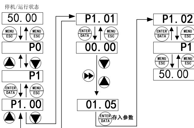
图3—2 三级菜单操作流程图
